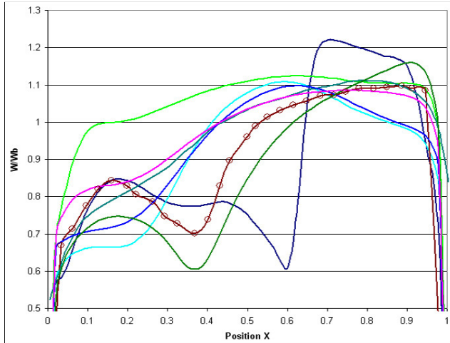
2a). Rake 2Y/D=0 on 90^\circ Plane
